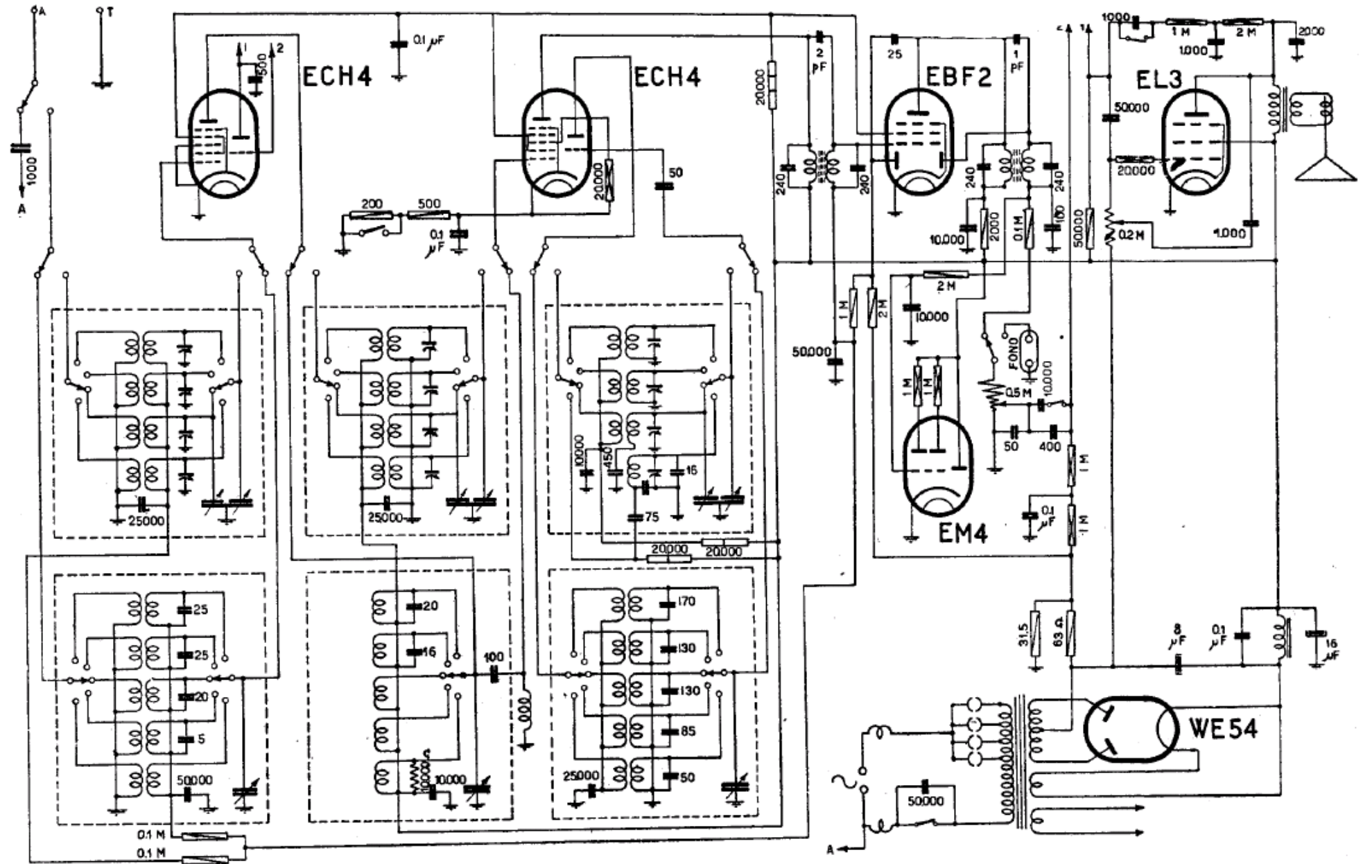
PHONOLA RADIO - Mod. 589 - Con due gruppi AF, uno per quattro gamme (da 150 a 320 kc, da 510 a 1580 kc, da 5,5 a 11,7 Mc, da 11 a 23 Mc) e l'altro per cinque bande allargate (16,3-17,2 m, 19,3-20,6 m, 24,4-26 m, 30-33 m, 46,2-52 m). Media frequenza 470 kc/s. Potenza d'uscita 4,5 W.
